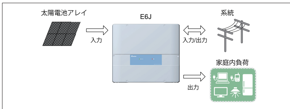
蓄電池切り離しモード
