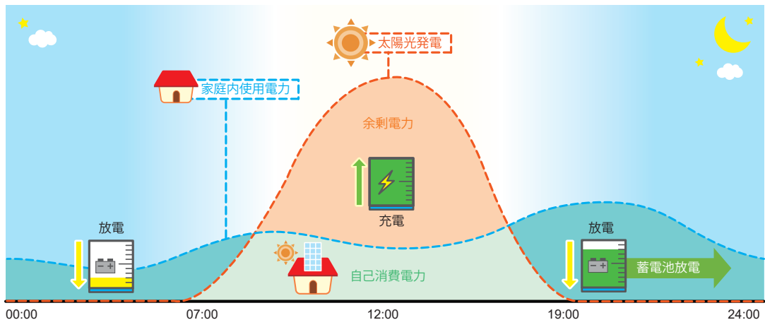
自家消費優先モードの動き
