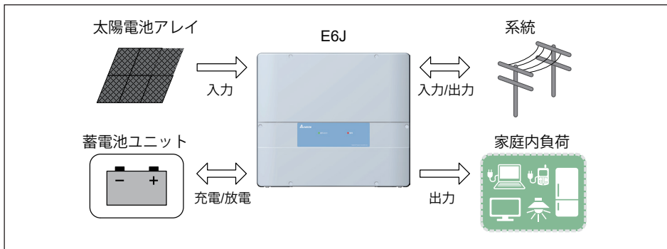
自家消費優先モード
